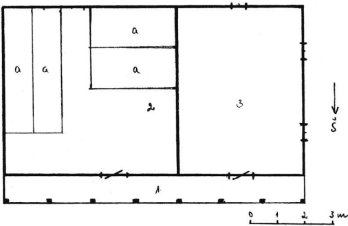
Medinė klėtis Steigvilių kaime, statyta XX a. pr. Klėties planas: 1 – prieklėtis, 2 – klėtis, 3 – klėtelė, a – aruodai
