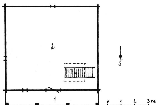
Klētis Bardiškių kaime, statyta 1928 m.
