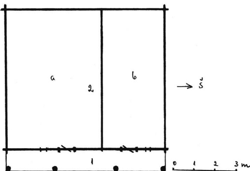
Klėtis Nakrošiūnų kaime, statyta 1881 m. (tašyti rąstai). Klėties planas: 1 – prieklėtis, 2 – klėtis a – didysis „skladas“, b – mažasis „skladas“
