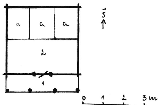
Klėtėlės planas:
