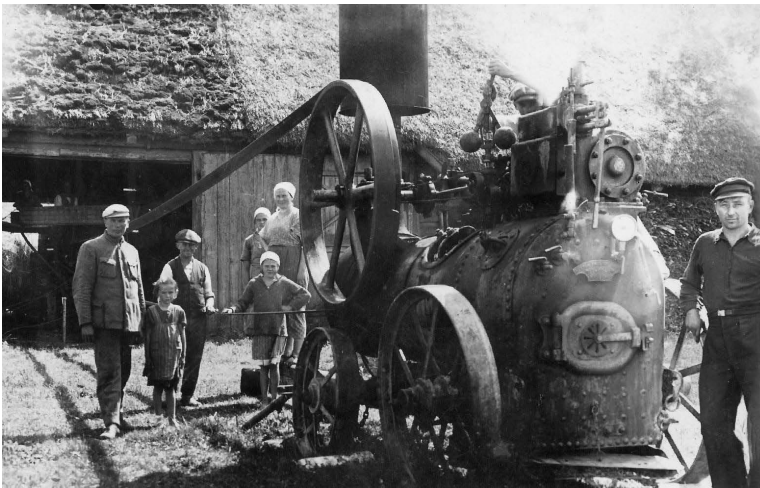
Lokomobilio varoma kuliamoji mašina prie daržinės
