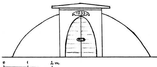
Rūsūs Bardiškių kaimo J. Kleinoto sodyboje, statytas 1933 m. J. Šliavo brėž.
